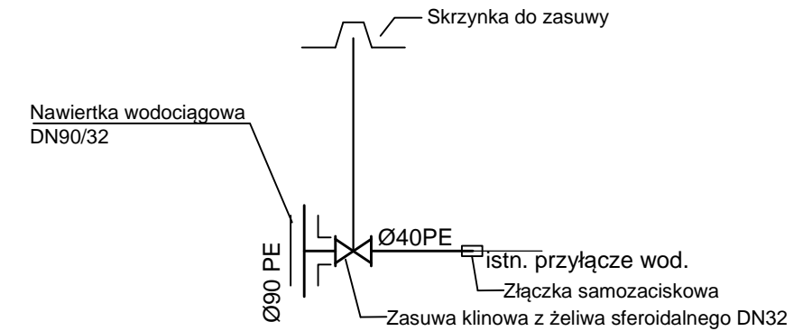
Przyłącza do posesji (Nr węzła: W2-W3)
