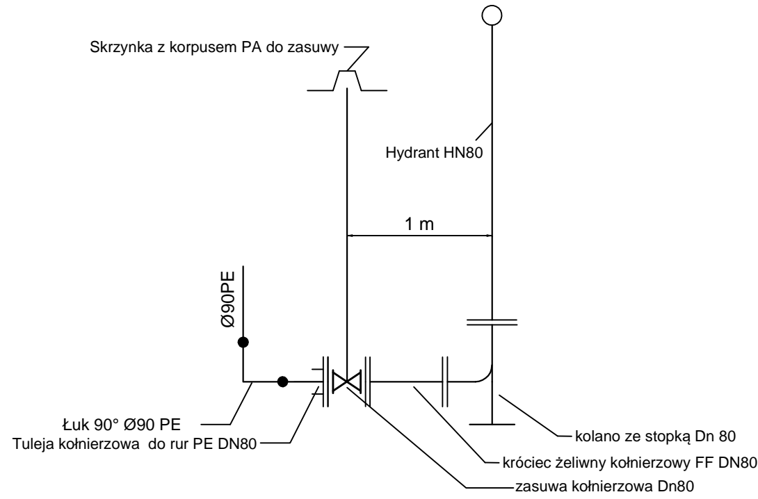
Węzeł hydrantowy nadziemny (Nr węzła: Hn1)
