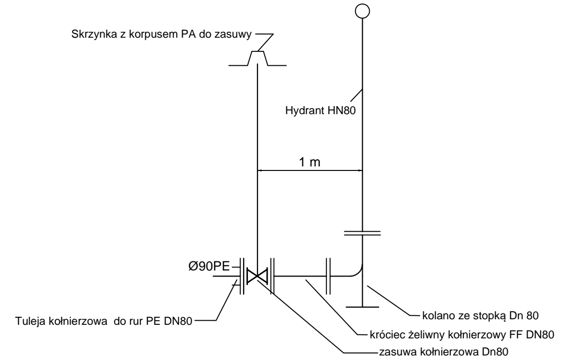
Węzeł hydrantowy nadziemny (Nr węzła: Hn2)
